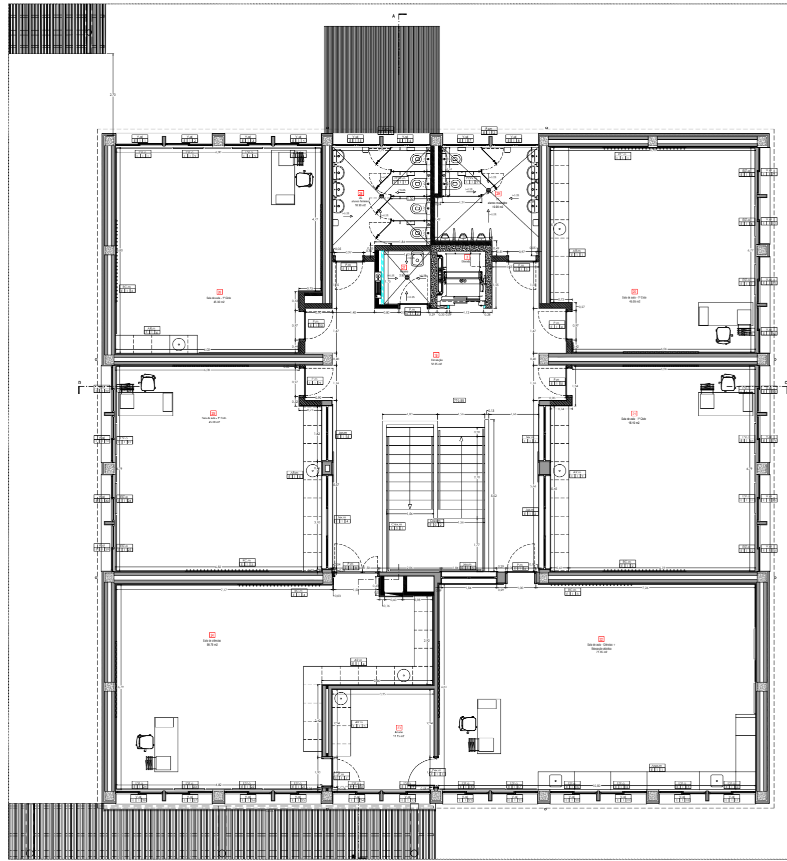
PLANTA DE PORMENOR DO PISO 1 - BLOCO 1 - ESC. 1/250
