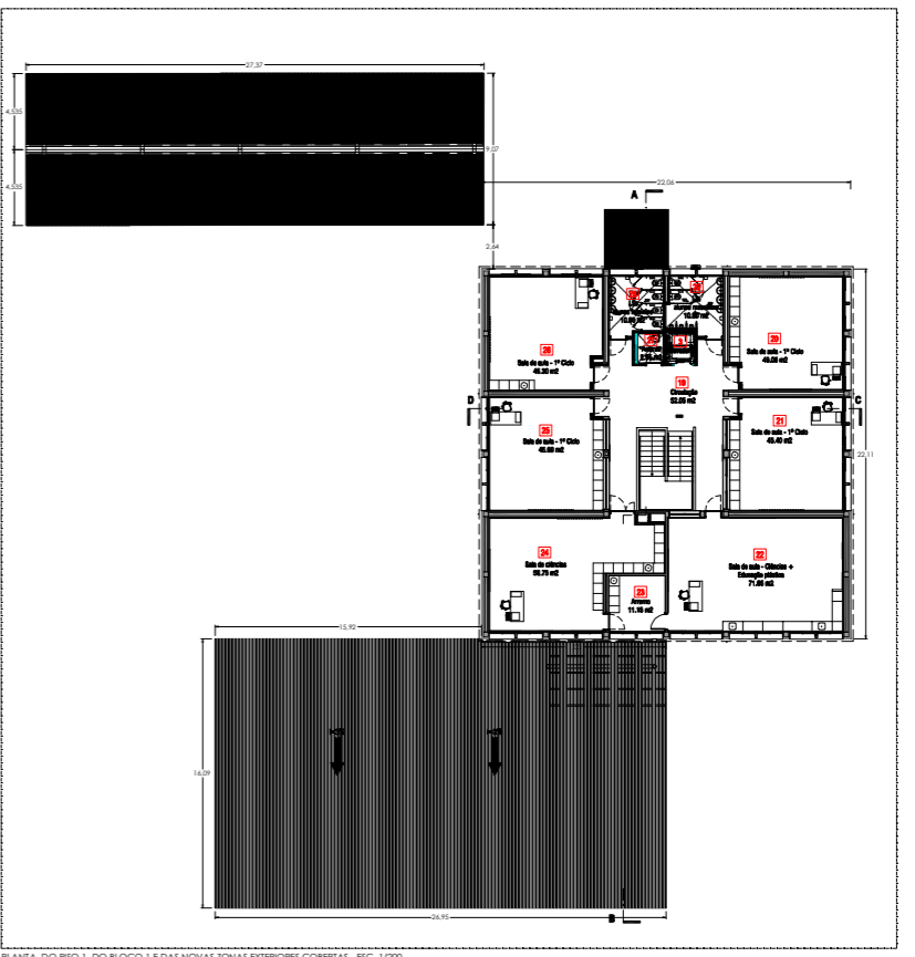
PLANTA DO PISO 1 DO BLOCO 1 E DAS NOVAS ZONAS EXTERIORES COBERTAS - ESC. 1/250
